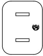
NEMA 1-15P
