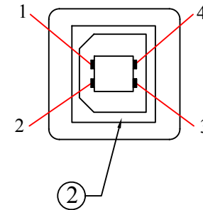
USB BF
